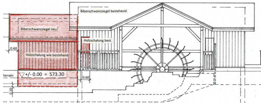
Projekt-Skizze Anbau
