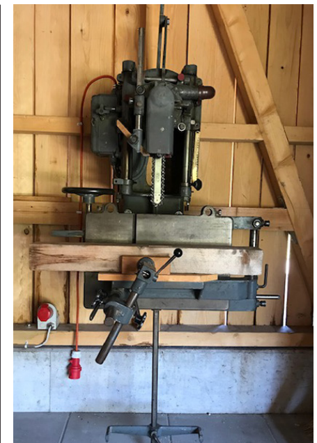
Kettenstemmer
